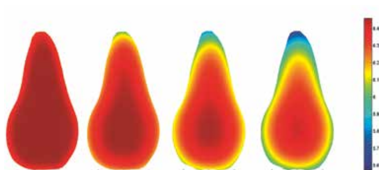
Figuur 3: Visualisatie van de waterconcentratie (% d.g.) in een peer, na 10 dagen bij 20°C en 75% R.V. (Vnr: dag 1, dag 4, dag 7, dag 10). Hierbij is duidelijk dat de peer aan de nek het meest uitdroogt.
